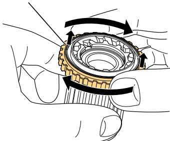
花鼓棘齿
