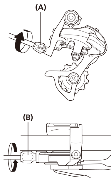
(А) Винт регулировки натяжения троса
