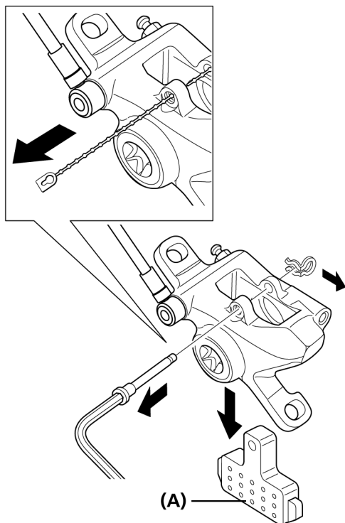
(A) Вкладыш для прокачки
