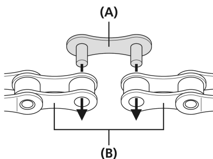
(A) Соединительное звено со штифтами
