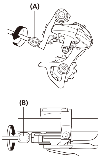
(А) Винт регулировки натяжения троса
