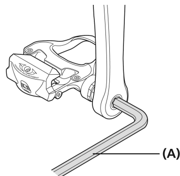
(A) Шестигранный ключ на 8 мм
