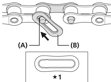
★1 Канавка должна быть обращена наружу
