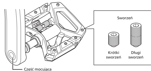
Bok pedału platformowego
