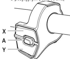
Zespół przełączników z przełącznikiem 3-pozycyjnym (lewa strona)
