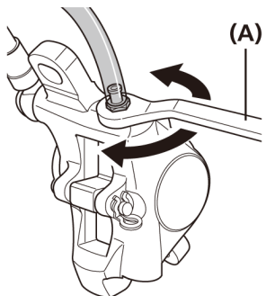
(A) Klucz oczkowy 7 mm
