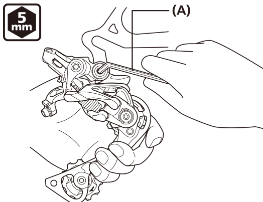
(A) Klucz imbusowy 5 mm
