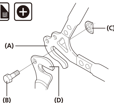
(A) Haki tylnego trójkąta (B) Śruba haka (C) Nakrętka haka (D) Hak
