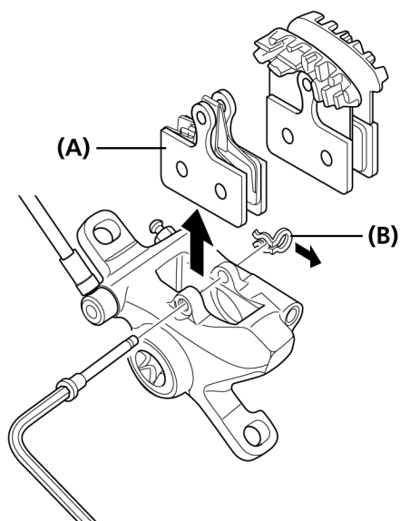
(A) Okładzina hamulcowa
