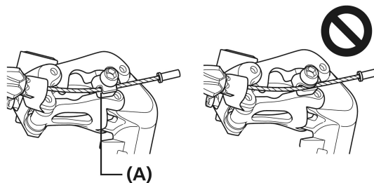
(A) Wyżłobienie
