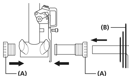
(A) Adapter (B) Mechanizm korbowy
