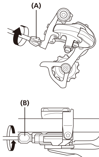
(A) Pokrętło regulacyjne linki
