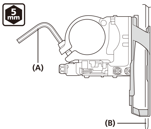
(A) Klucz imbusowy 5 mm (B) Największa tarcza
