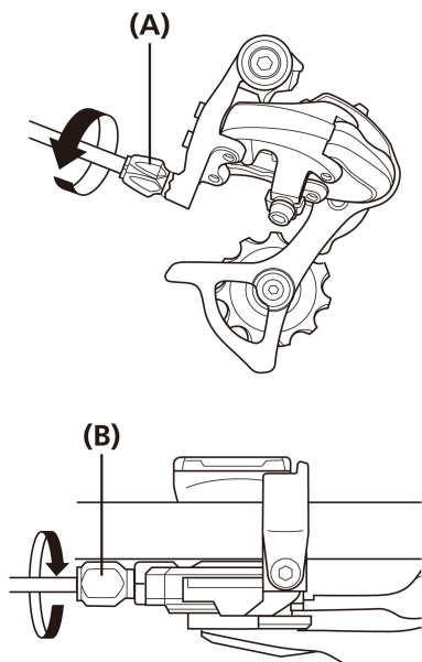
(A) Pokrętło regulacyjne linki
