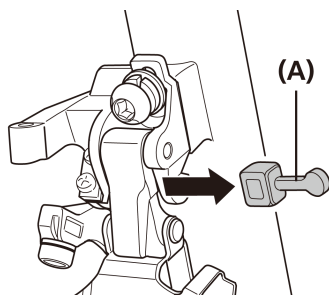
(A) Blokada regulująca Pro-Set
