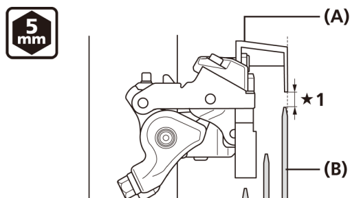
(A) Klucz imbusowy 5 mm (B) Największa tarcza
