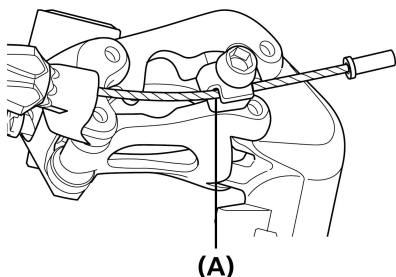
(A) Wyżłobienie
