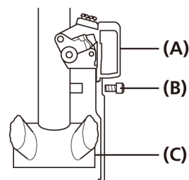
(A) Przerzutka przednia (B) Śruba (C) Położenie osi suportu
