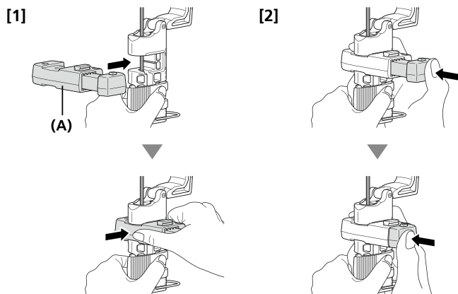
(A) Obcinak do przewodów
