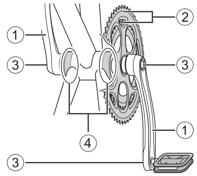
비유니트 베어링의 경우 / 使用非軸承組件時
