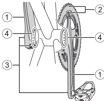
유니트베어링케이스 안에 / 使用軸承組件時
