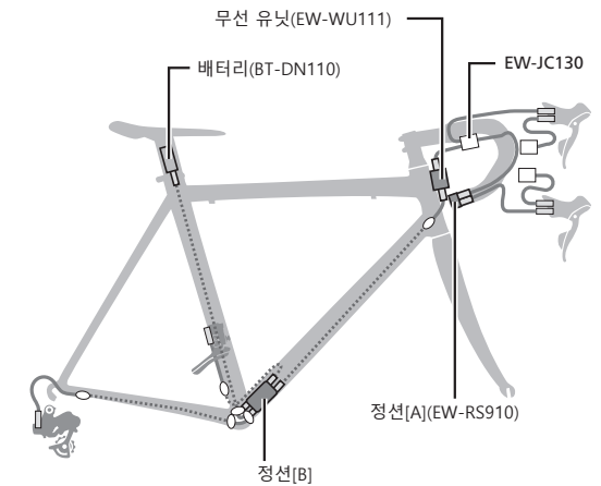
EW-WU111/EW-RS910(내장형 바랜드 타입)
