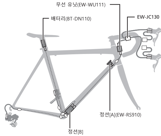
EW-WU111/EW-RS910(내장형 프레임 타입)
