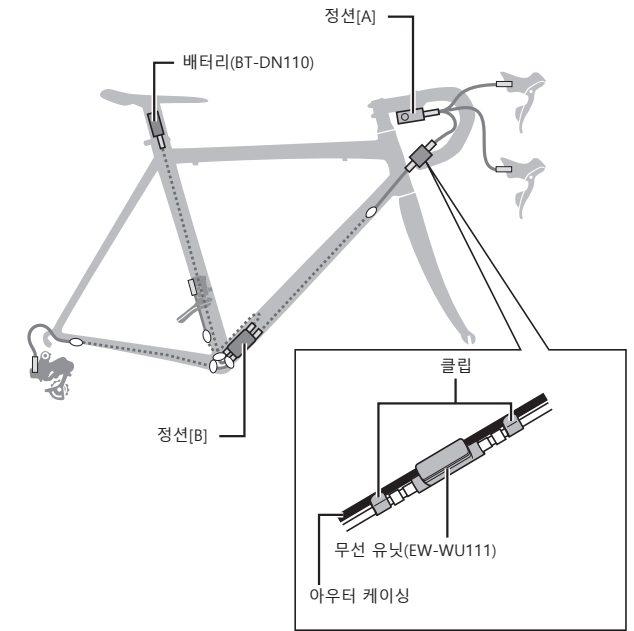
EW-WU111/EW-RS910(내장형 바랜드 타입)
