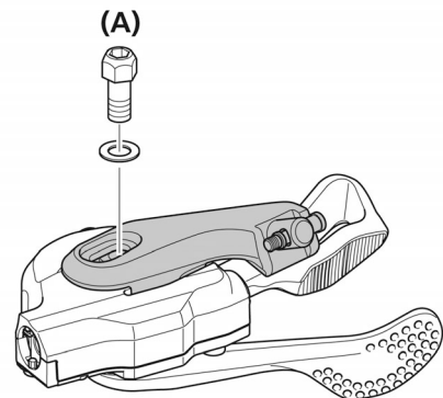
(A) 유닛 고정 볼트(I-spec B)
