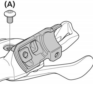
(A) 유닛 고정 볼트(I-spec II)
