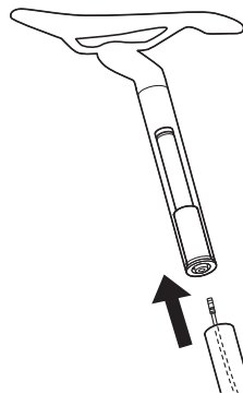
배터리 마운트용 일렉트릭 와이어 [내장형 배터리인 경우(SM-BTR2/ BT-DN110/BT-DN110-A)]
