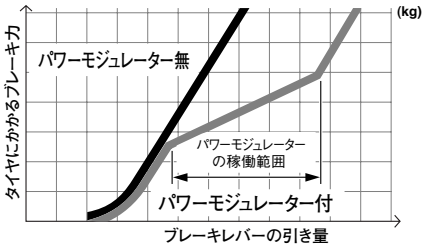
パワーモジュレーターのブレーキ性能
