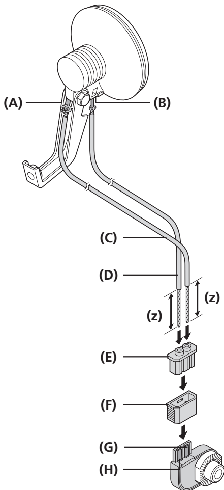
ハブダイナモの接続ターミナル
