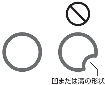
クランプバンドを固定する ハンドルバーの断面図
