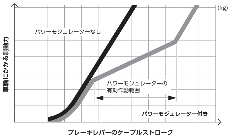
制動性能の比較
