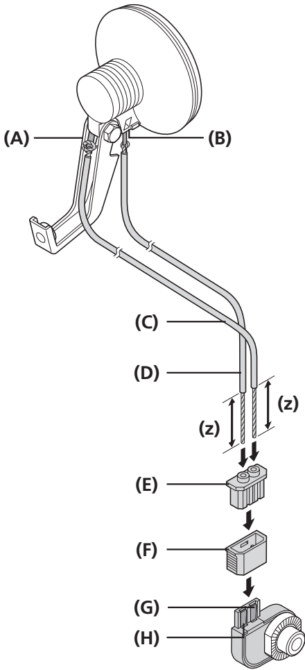
ハブダイナモの接続ターミナル
