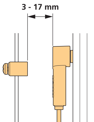
スピードセンサーと磁石ユニットの距離
