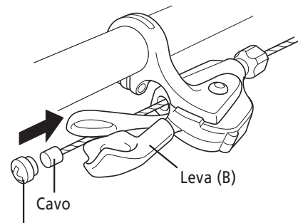
Cappuccio dell'ancoraggio dell'estremità del cavo
