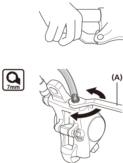
(A) Chiave combinata da 7 mm
