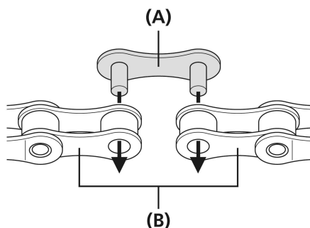
(A) Maglia di connessione con perni (B) Maglia interna
