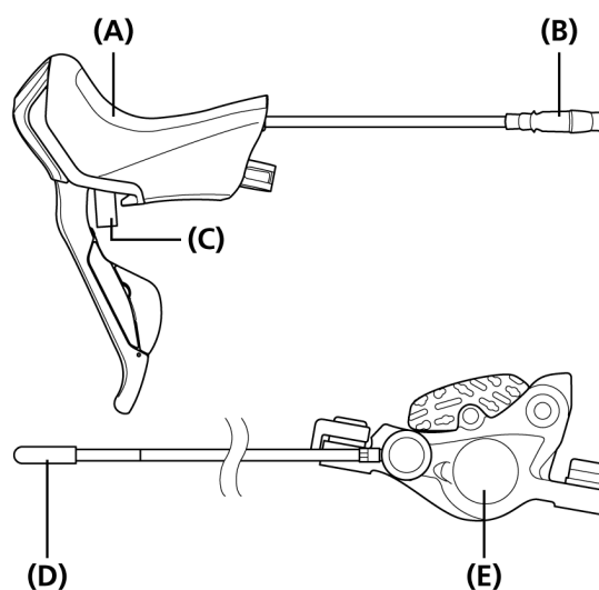
(A) Leva Dual control (B) Manicotto di giunzione (C) Stopper della leva (D) Cappuccio tubo (E) Pinza freno
