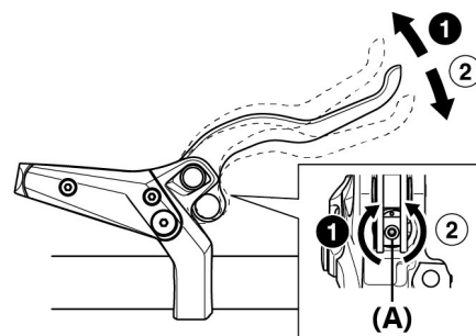
(A) Perno di regolazione dell'escursione
