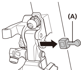
(A) Dispositivo di allineamento Pro-Set
