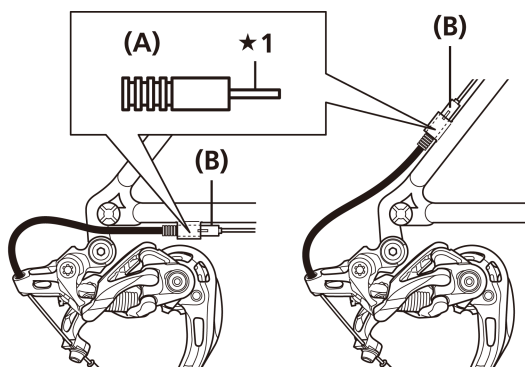
(A) Capoguaina sigillato con linguetta
