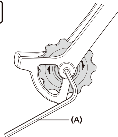
(A) Brugola da 3 mm
