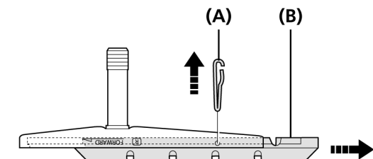
(A) Perno di fissaggio del pattino (B) Pattino
