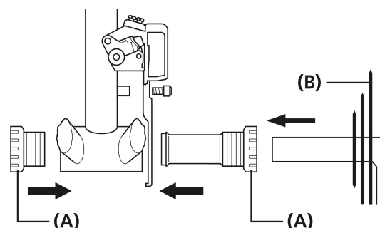
(A) Adattatore (B) Corona
