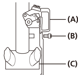
(A) Deragliatore (B) Bullone (C) Posizione del movimento centrale
