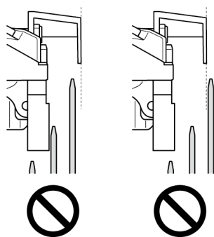
(A) Piastrina esterna del guidacatena (B) Corona più grande
