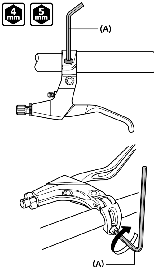
(A) Brugola da 4 mm/5 mm
