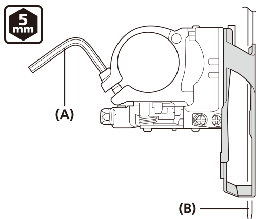
(A) Brugola da 5 mm (B) Corona più grande
