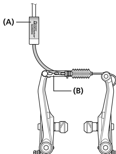
(A) Modulatore di potenza
