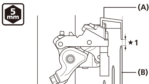
(A) Brugola da 5 mm (B) Corona più grande
