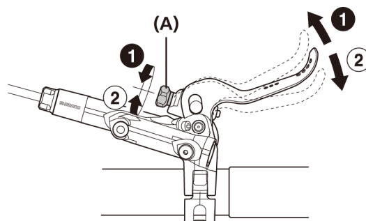
(A) Perno di regolazione dell'escursione
