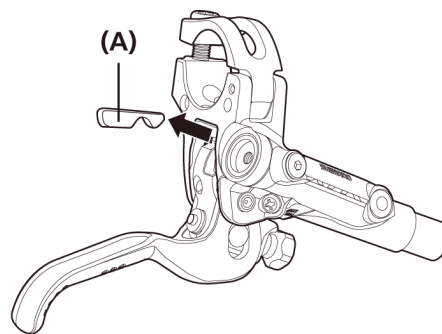
(A) Stopper della leva
