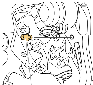
Goupille de butée de plaque
