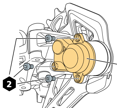
Cache de l'unité de plaque
