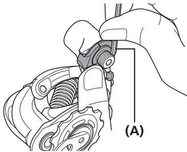
(A) Llave hexagonal de 3 mm
