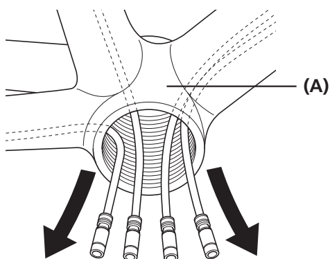
Cable eléctrico para el soporte de la batería [En el caso de una batería externa (SM-BTR1)]
