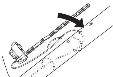
Cable eléctrico para el soporte de la batería [En el caso de una batería externa (SM-BTR1)]
