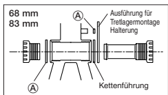
(A) : 2,5 mm Zwischenscheibe
