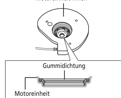
Motoreinheit innen
