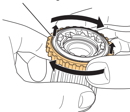
Nabenverzahnung
